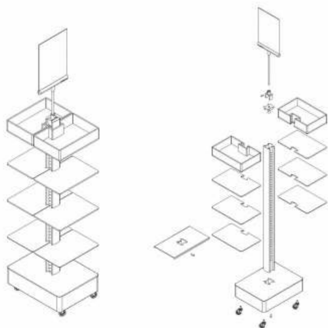
型号(Item No.): FLD-SJ1 高度(Height) : 1650mm
