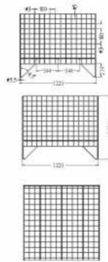
型号(Item No.): FLD-DB10
